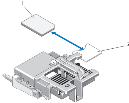
Rakam 14. SD vflash kartını deęiřtirme
