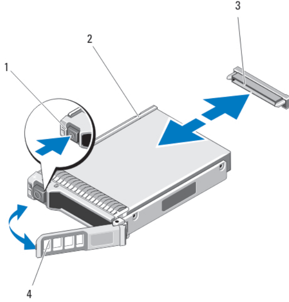
Rakam 19. Sabit Sürücüyü/SSD'yi Çıkarma ve Takma
