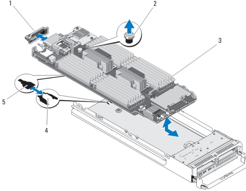
Rakam 22. Sistem Kartını Çıkarma ve Takma
