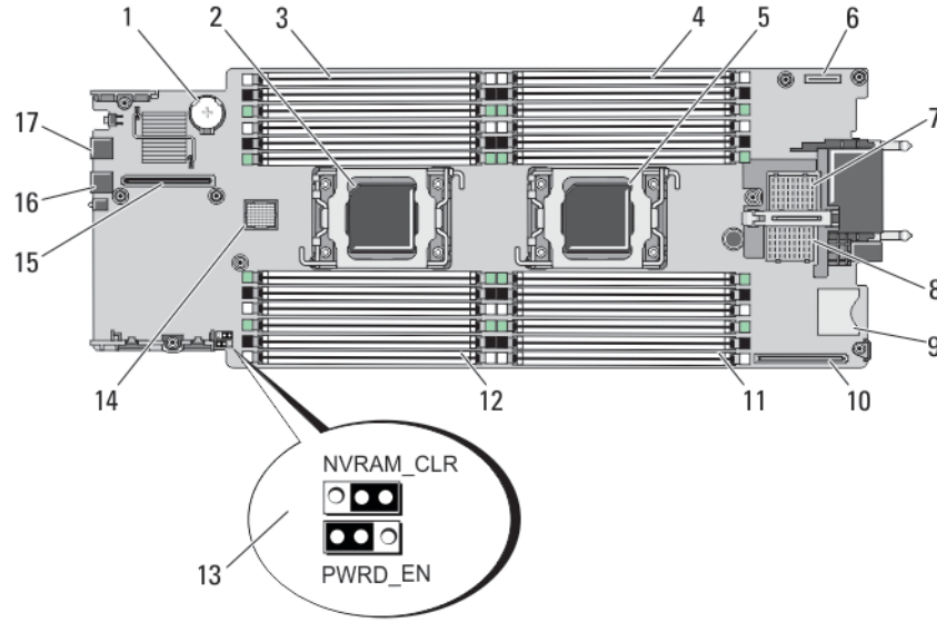
Rakam 25. Sistem Kartı Konektörleri
