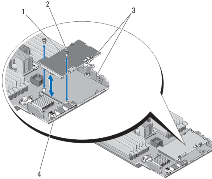
Rakam 24. Depolama Denetleyicisi Kartının Çıkarılması ve Takılması
